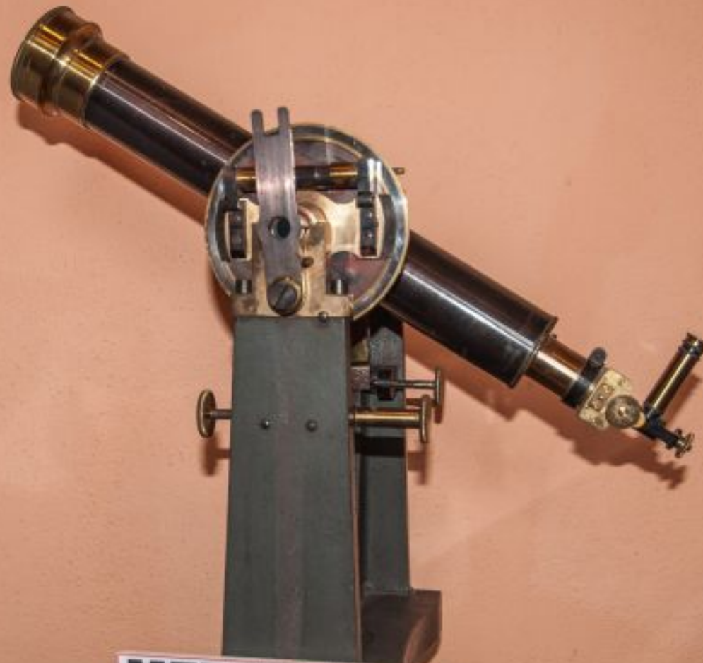
MERIDIENNE UTILISEE AUTREFOIS POUR MESURER AVEC PRECISION LA POSITION DES ASTRES GAD GROUPE D'ASTRONOMIE
