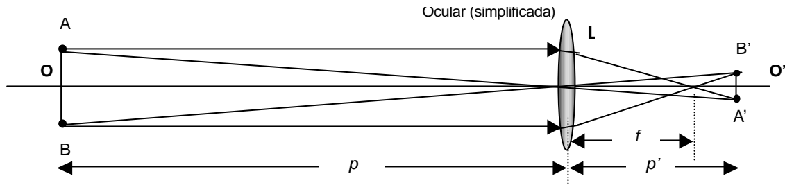
Fig. 5.- A partir do orifício O, bem iluminado (de diâmetro \overline{AB} ), a ocular L forma a imagem reduzida O' (diâmetro \overline{A'B'} = y ), localizada um pouco além do diafragma de campo dessa ocular (Fig. 6). É esta imagem reduzida do orifício O que será a nossa estrela artificial.
