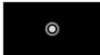
Fig. 9.- Figura de difracção típica, observável com um telescópio com 33% de obstrução (amplificação de cerca de 2,4x por milímetro de abertura). Num telescópio sem obstrução (refractor), o primeiro anel de difracção é mais tênue.
