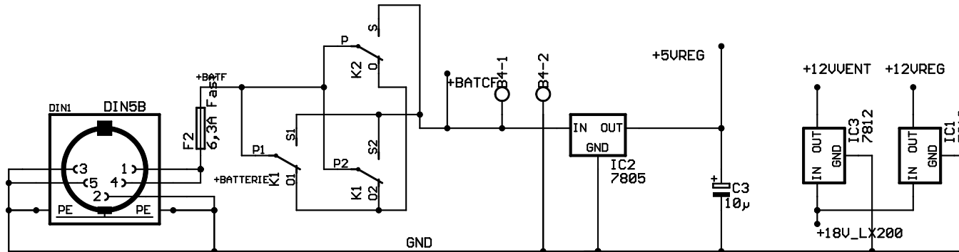
Batterie 12U
